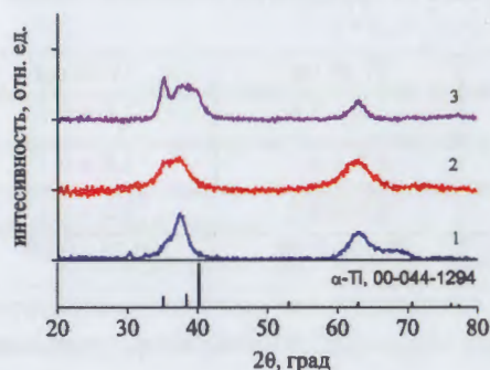
Рисунок 7. Дифрактограммы, полученные для пленок Ti: 10 нм (1), 20 нм (2) и 60 нм (3).
