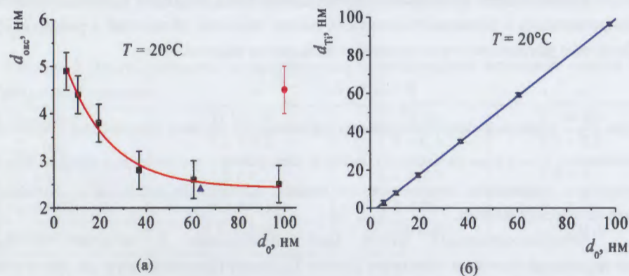
Рисунок 2. Зависимости толщины оксидного слоя d_{\text{окс}} (а) и толщины неокисленного слоя титана d_{\text{Ti}} (б) в бислойной структуре Ti/TiO 2 от исходной толщины окисляемой титановой пленки d_0 . Цветными символами на рис. 2 (а) обозначены толщины оксидных слоев, полученных при окислении: \blacktriangle – пленки ультрачистого Ti толщиной 63.5 нм [10]; \bullet – пленки Ti толщиной 100 нм [11].
