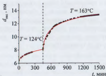
Рисунок 4. Кинетическая кривая окисления пленки Ti толщиной 40 нм, полученная путем измерения ее электрического сопротивления
